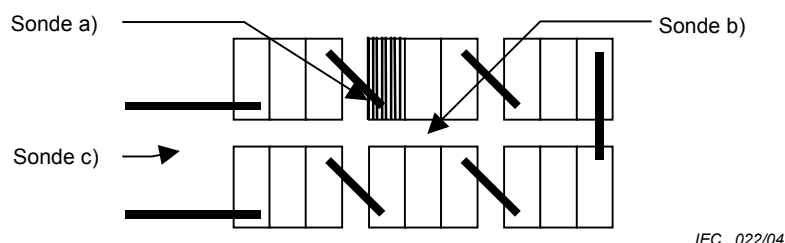
Figure 7 – Vue de dessus de l'installation pour des éléments et batteries monoblocs
