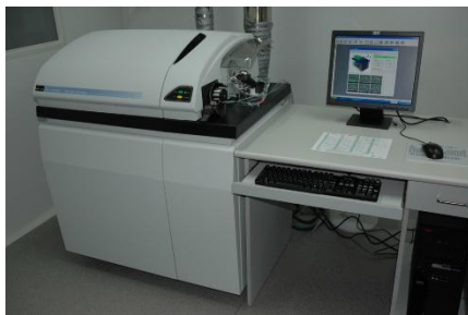
•ICP-MS
